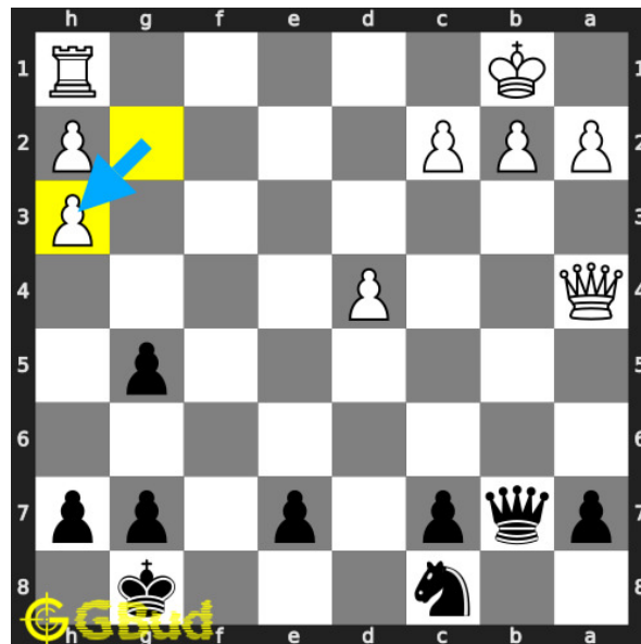
Figure 4: g3h3
